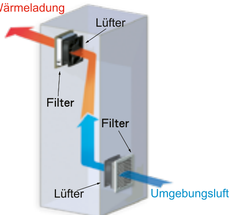
Abb.2 Abluft mit Überdrucksystem
