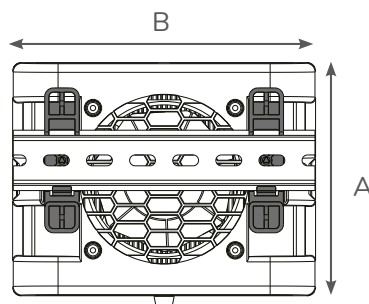
TG 3039303 DIN Schienenmontage
