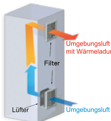
Abb.3 Überdrucksystem
