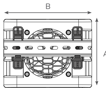
TG 3039309 DIN Schienenmontage
