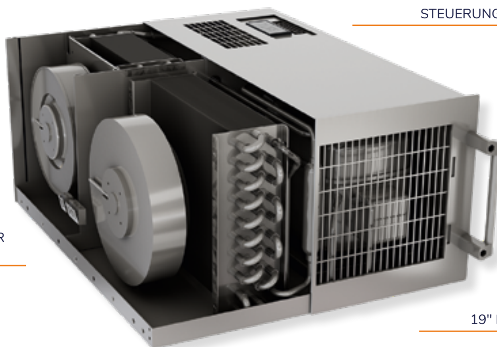
Abb. Kompressorkühlgerät 19"
