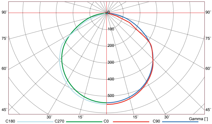
Lichtverteilungskurve
